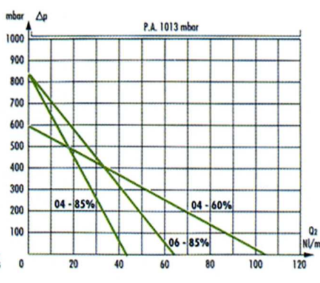
Niveau de vide (mbar) en fonction du débit (NI/min)
